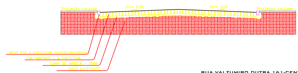
03 PERFIL TRANSVERSAL ESCALA: 1/75
