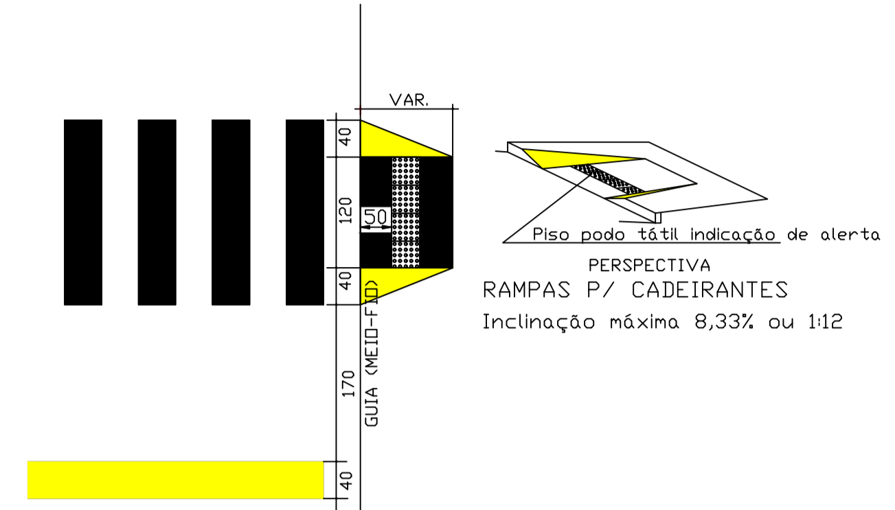
05 DETALHAMENTO FAIXA DE PEDESTRES E RAMPAS S/E
