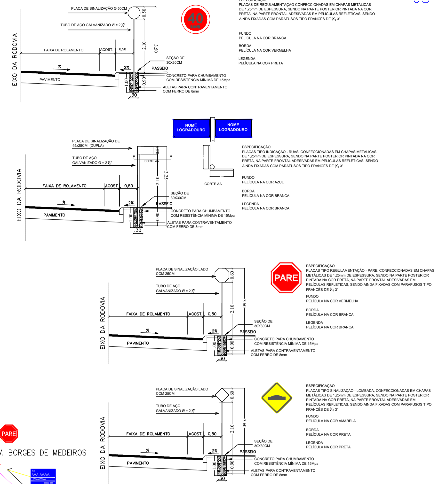
04 DETALHAMENTO SINALIZAÇÃO VERTICAL S/E
