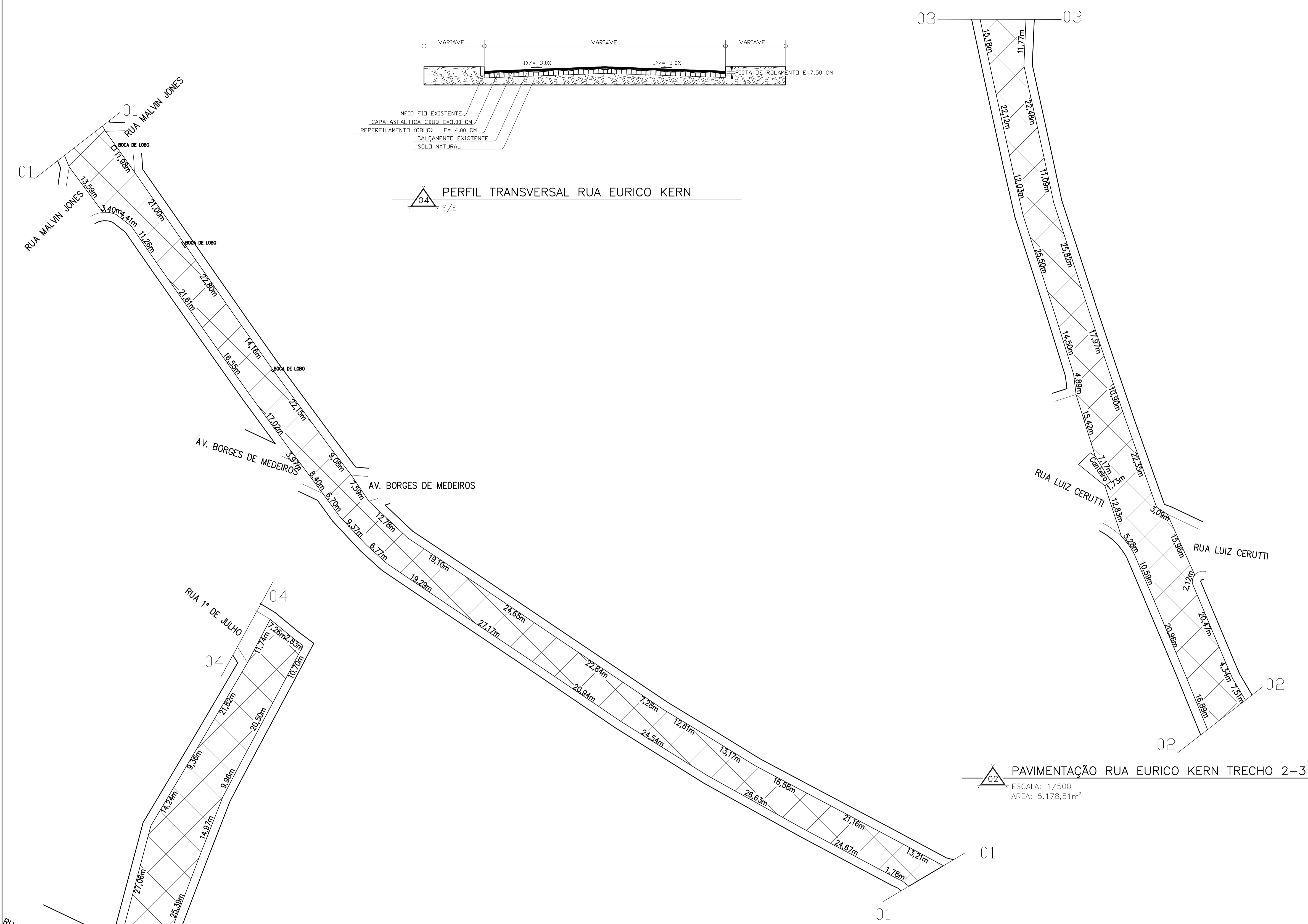
01 ESCALA: 1/500 ÁREA: 5.178,51m 2 PAVIMENTAÇÃO RUA EURICO KERN TRECHO 1-2
