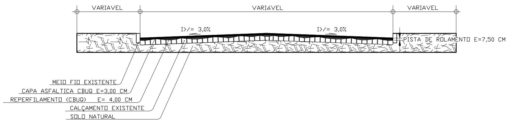
04 S/E PERFIL TRANSVERSAL RUA EURICO KERN
