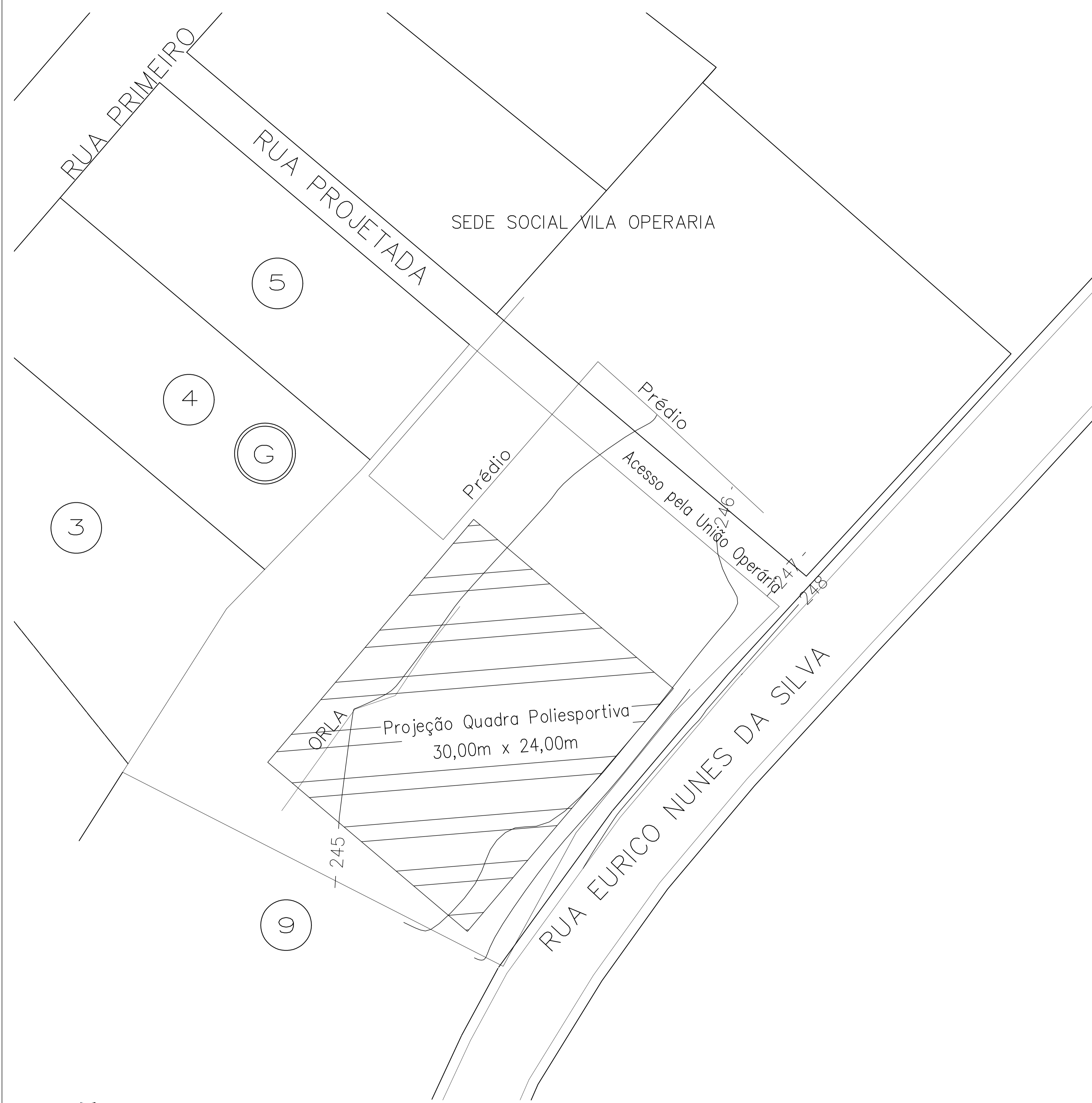
PLANTA_SITUACAO_E_LOCALIZACAO ESCALA: 1:200
