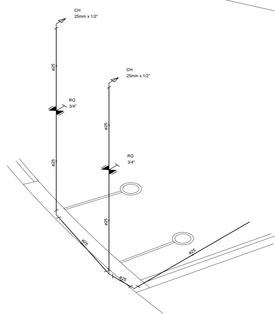
Detalhe Chuveirinho escala 1:25
